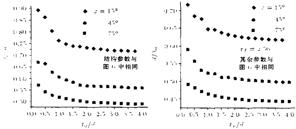
(a) 第一次强烈反射频率随周期层厚度的变化曲线
