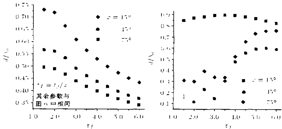
(a) 第一次强烈反射频率随周期层厚度的变化曲线
