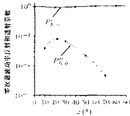
图2 零次空间谐波功率反射系数 随水平入射角度的变化曲线
