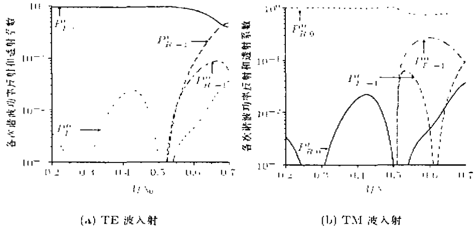
图 4 各次空间谐波反射和透射特性随频率的变化曲线
