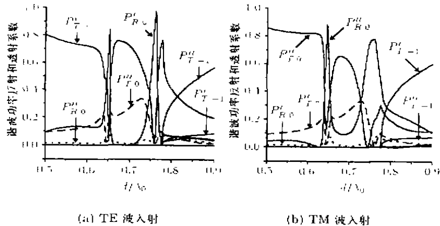
图 5 各次空间谐波反射和透射特性随频率的变化曲线
